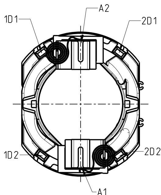
Ansicht von der Kollektorseite
